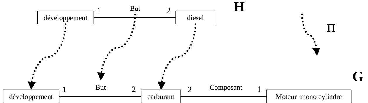
Fig. 5 – Exemple de pseudo-projection de H dans G .
