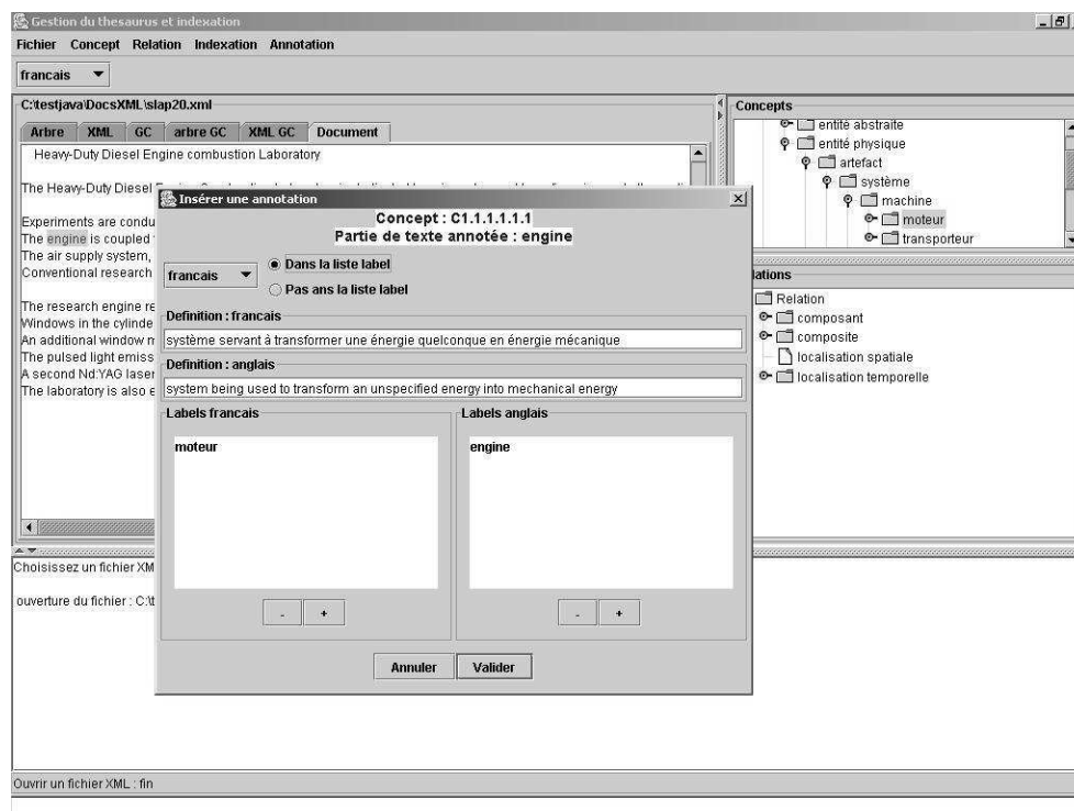
Fig. 10 – Le module d'annotation de SYDOM
